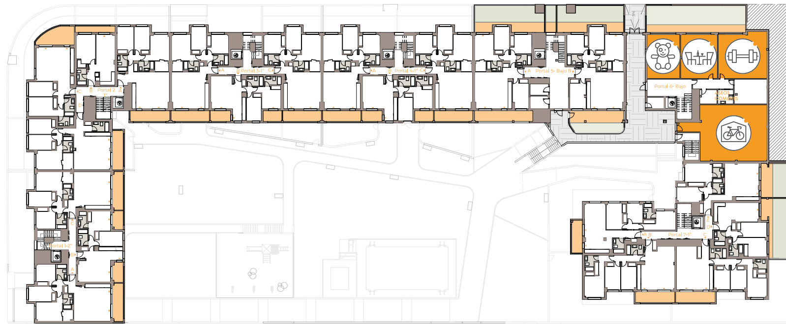
PLANTA BAJA
